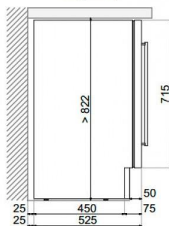
Вид сбоку
