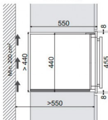
Вид сбоку
